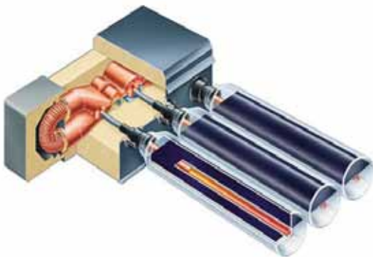
Abb.3: Vakuumröhrenkollektor
