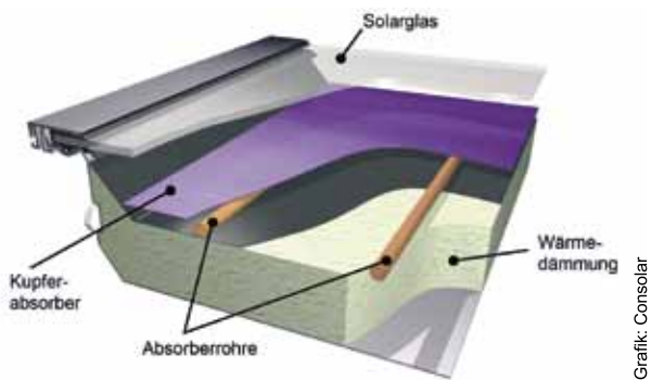
Abb.2: Aufbau eines Flachkollektors
