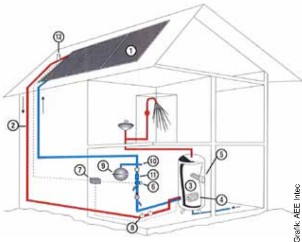
Abb. 1: Solaranlage schematisch
